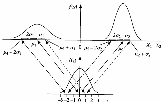
Fig. 2 – Funzioni di densità di variabili casuali normali rese standard
